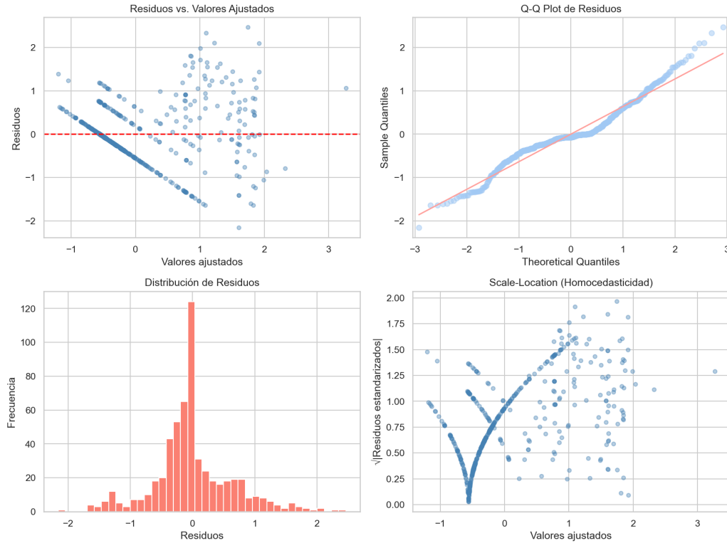
Figura 3.2: Gráficos de diagnóstico del modelo OLS. Superior derecha: Q-Q plot de residuos, con ajuste razonable a la línea teórica salvo en los extremos. Inferior izquierda: distribución de residuos aproximadamente simétrica. Ambos gráficos sugieren que la desviación de normalidad no compromete la inferencia.
