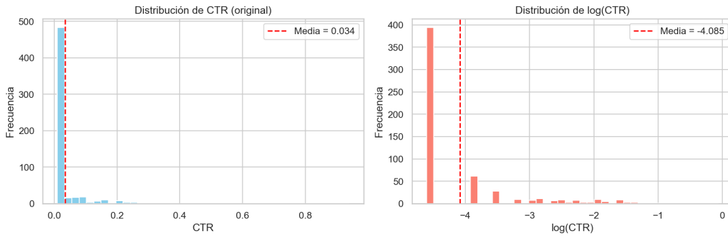
Figura 3.1: Distribución del CTR original (izquierda) y de \log(\text{CTR}) (derecha). La transformación logarítmica reduce la asimetría de 6,78 a 1,87 y elimina la cola derecha extrema, haciendo la distribución más apta para el modelo OLS. El pico visible en \log(\text{CTR}) \approx -4,6 corresponde al valor mínimo reportado de \text{CTR} = 0,01 ( floor effect ).
